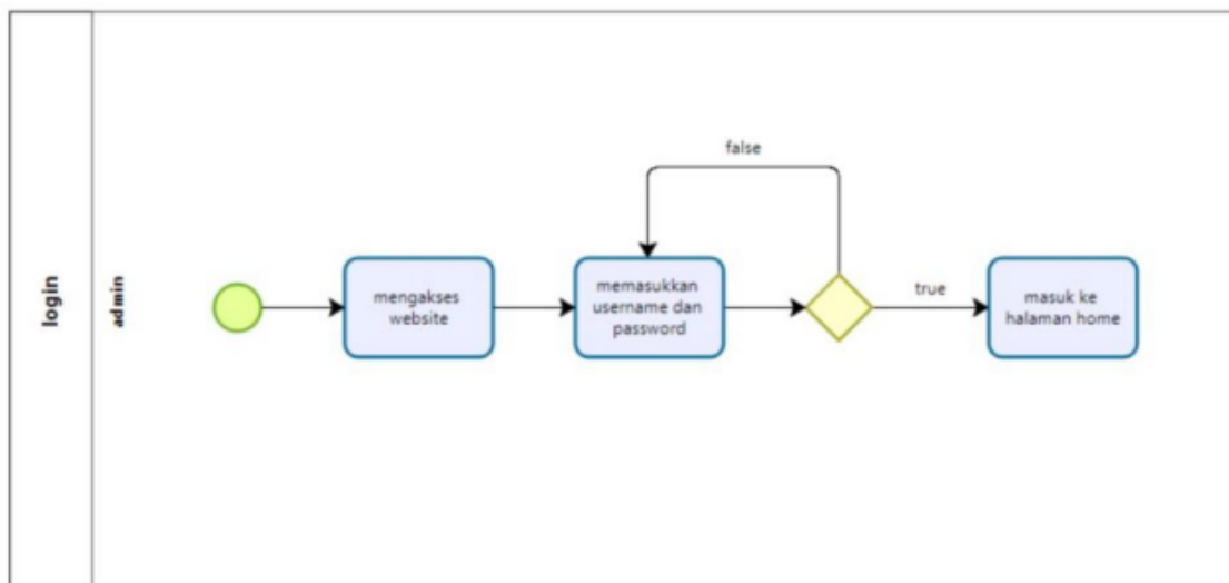
Gambar 3 BPMN Login
